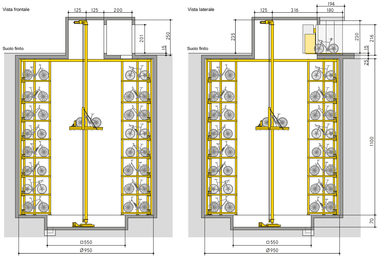
Sezione livello di parcheggio
