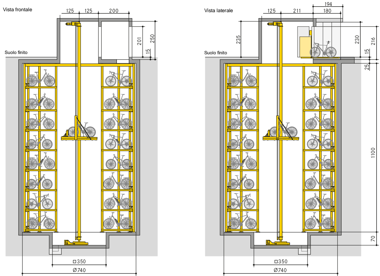
Sezione livello di parcheggio
